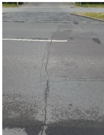
Abbildung 33 Rissbildung in der Fahrbahndecke
